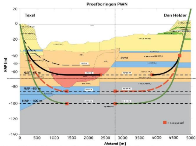
Figuur 1.3 Schematisch dwarsproef met de proefboorlijnen; (bochten van boorlijnen niet op schaal).
